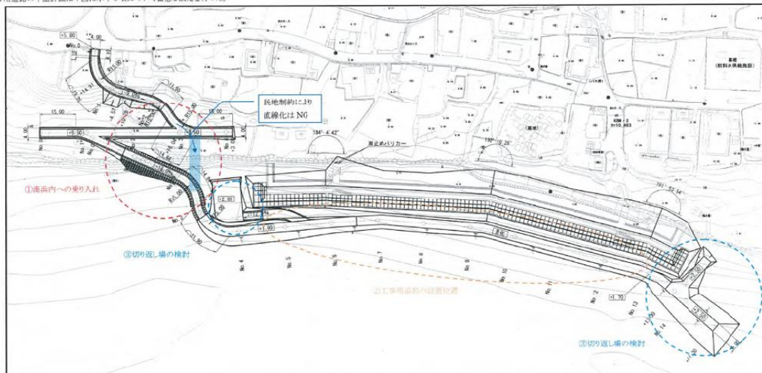
図 2.3.3 工事用道路平面図
